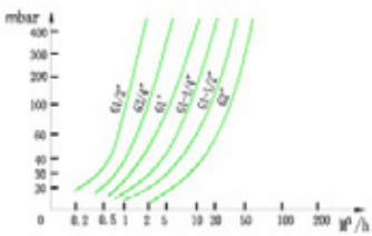
График 2 – Зависимость потерь давления от расхода
