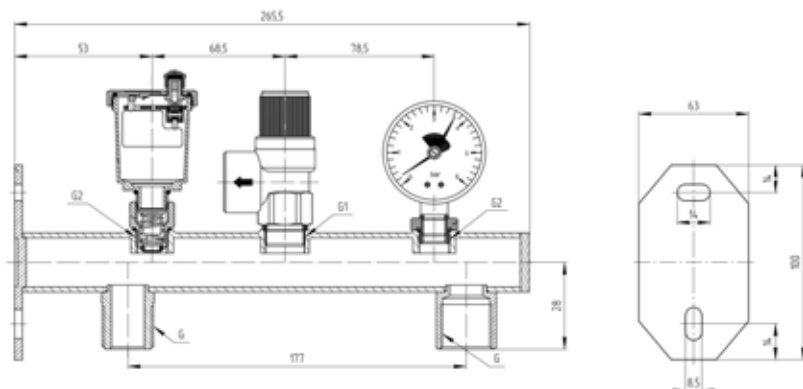
Рисунок 2 – Габаритные размеры.
