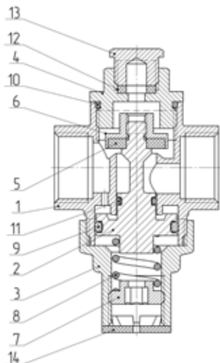
Рисунок 2 – Конструкция регулятора
