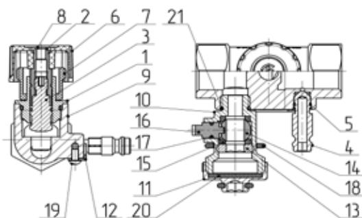
Рисунок 2 – Конструкция клапана
