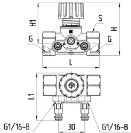
Рисунок 3 – Габаритные размеры клапана.
