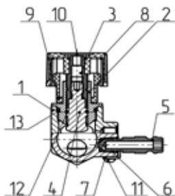
Рисунок 2 – Конструкция клапана
