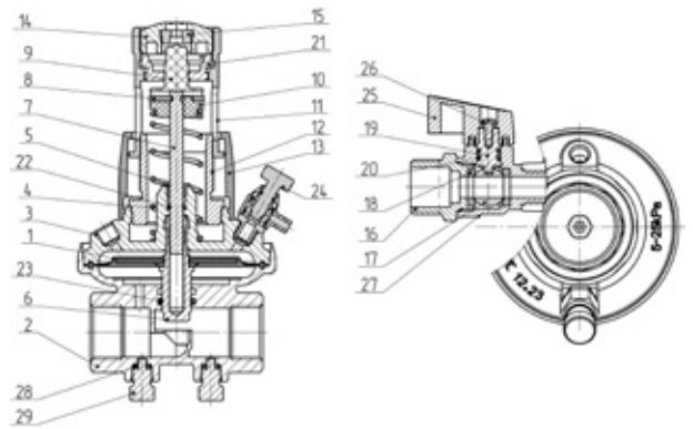
Рисунок 2 – Конструкция клапана
