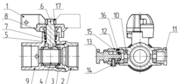
Рисунок 1 – Конструкция шарового крана
