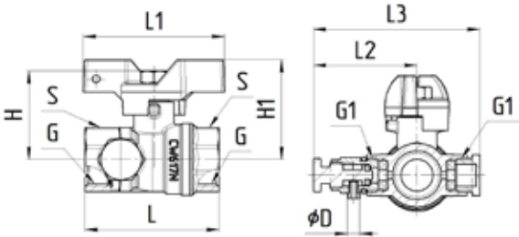
Рисунок 2 – Габаритные размеры крана.
