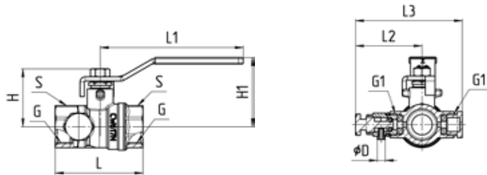
Рисунок 2 – Габаритные размеры крана.
