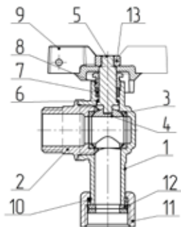
Рисунок 1 – Конструкция шарового крана
