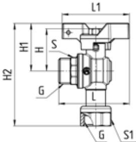
Рисунок 2 – Габаритные размеры крана.
