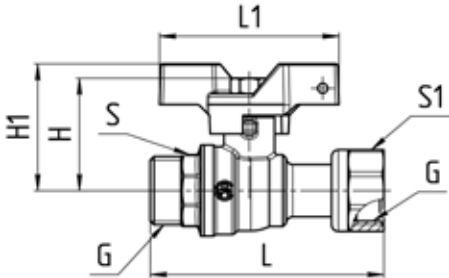
Рисунок 2 – Габаритные размеры крана.
