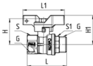
Рисунок 2 – Габаритные размеры крана.
