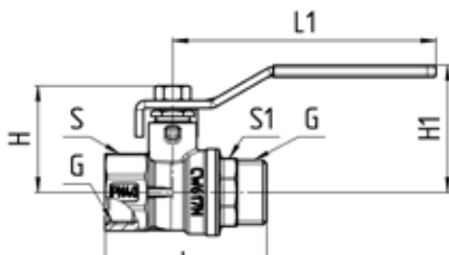
Рисунок 2 – Габаритные размеры крана.
