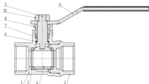
Рисунок 1 – Конструкция шарового крана
