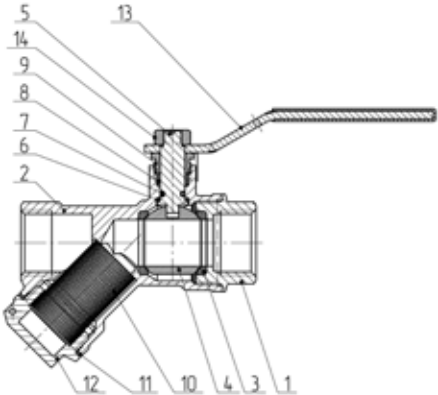
Рисунок 1 – Конструкция шарового крана
