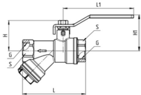
Рисунок 2 – Габаритные размеры крана.
