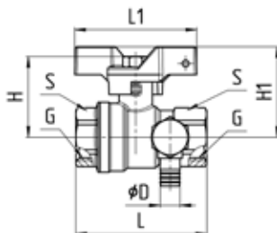
Рисунок 2 – Габаритные размеры крана.
