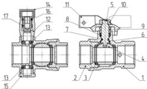
Рисунок 1 – Конструкция шарового крана со спускником
