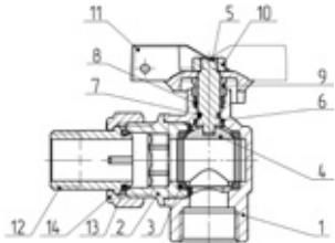
Рисунок 1 – Конструкция шарового крана
