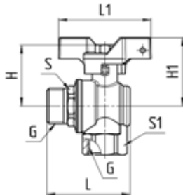
Рисунок 2 – Габаритные размеры крана.
