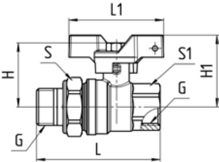
Рисунок 2 – Габаритные размеры крана.
