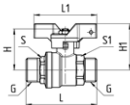
Рисунок 2 – Габаритные размеры крана.
