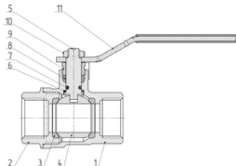
Рисунок 1 – Конструкция шарового крана
