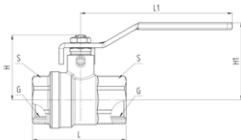
Рисунок 2 – Габаритные размеры крана.
