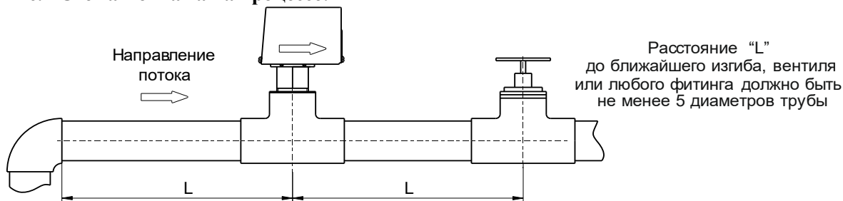
Рис.4 Схема монтажа на процессе:
